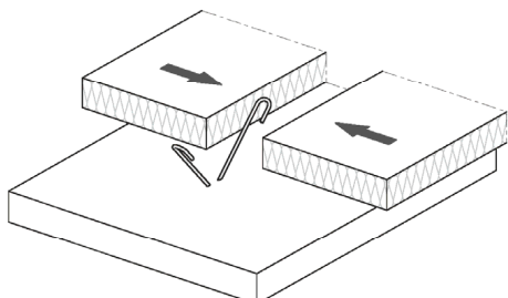
Bild 17: Geteilte Dämmstoffplatte seitlich am Anker zusammenschieben.
