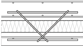
Bild 23: Bewehrung der oberen Schicht einbauen, Zusatzbewehrung entsprechend Anlage 4, Tabelle 2, durch die Bügelenden der Traganker durchstecken und befestigen. Einbindetiefen der Anker gemäß Anlage 4, Tabelle 2, einhalten.
