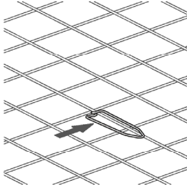
Bild 9: Verbundbügel unter den oberen Mattenstab führen.
