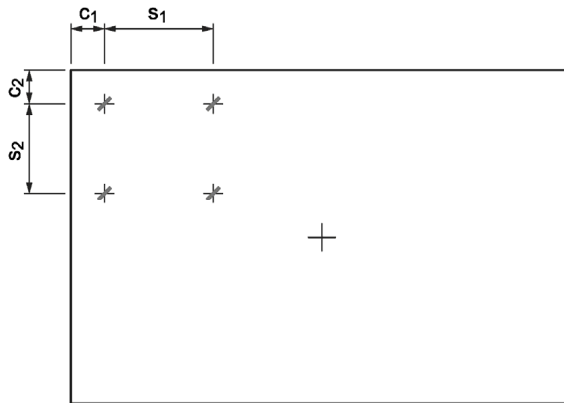
Rand- und Achsabstände der Verbundanker
