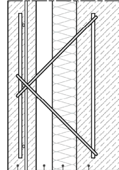
Sandwichanker Typ 1 / Typ 2 (Beispiel Vierschicht-Platte)
