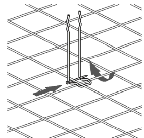
Bild 8: Anstecknadel um den oberen Mattenstab führen und senkrecht aufstellen. Danach mit Nagel oder Stift fixieren.
