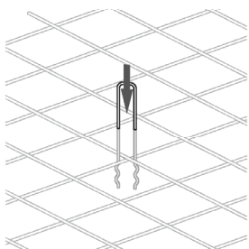
Bild 19: Verbundnadel spätestens 60 min. nach Zugabe des Anmachwassers durch die Dämmstoffplatte in den Frischbeton bis zum Schalungsboden drücken. Danach die Verbundnadel bis zum Erreichen der erforderlichen Einbindetiefe wieder herausziehen. Ein Eintragen der Wärmedämmung in den Verankerungsgrund ist zu verhindern.
