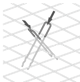
Bild 20: Verbundnadeln spätestens 60 min. nach Zugabe des Anmachwassers nacheinander unter 45° durch die Dämmstoffplatte in den Frischbeton bis zum Schalungsboden drücken. Der Kreuzungspunkt der beiden Nadeln soll in der Mitte der Wärmedämmung liegen. Danach die Verbundnadeln bis zum Erreichen der erforderlichen Einbindetiefe wieder herausziehen.
