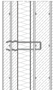
Verbundnadelkreuz VNK (Beispiel Dreischicht-Plate)
