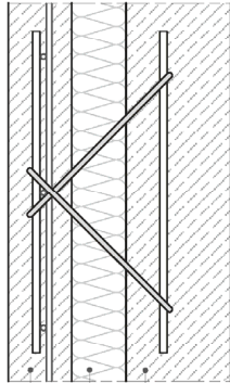
Sandwichanker Typ 1 / Typ 2 (Beispiel Dreischicht-Platte)
