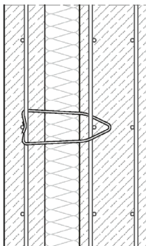
Verbundbügel VB (Beispiel Dreischicht-Plate)
